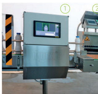
Weight and cap monitoring system (1) with an automatic rejection device (2) Устройство для проверки точности дозирования и наличия крышек
